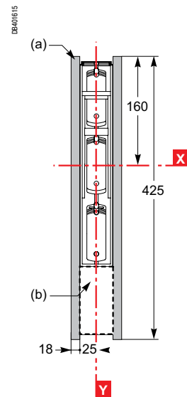
Держатель плавких вставок разомкнут и заблокирован
