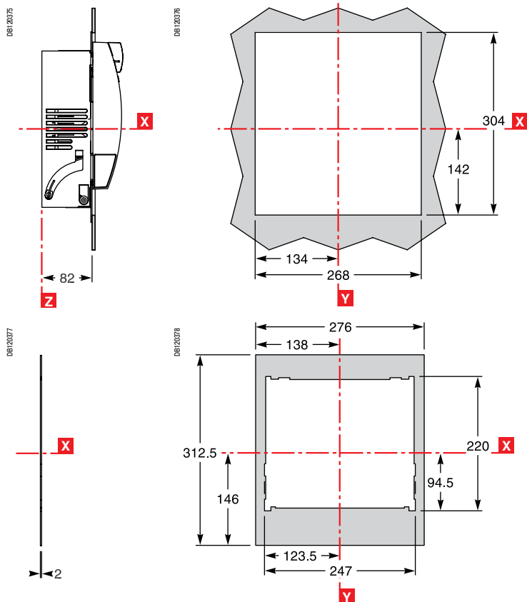
Вырез для 1 устройства
