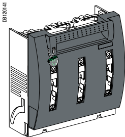
Опломбирование аппаратов SFT100 - ISFT630
