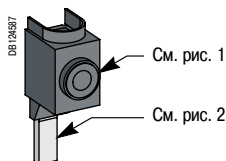
Входная клемма для гребенчатых шин
