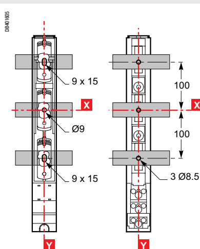
Для 100 мм шин
