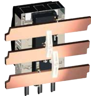
ISFT160 (нажимное присоединение)
