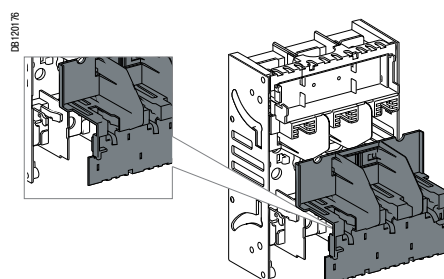
Размещение блока контактов сигнализации срабатывания предохранителей
