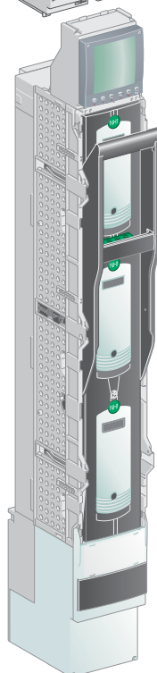
ISFL 250-630 + пластиковая коробка Power Meter
