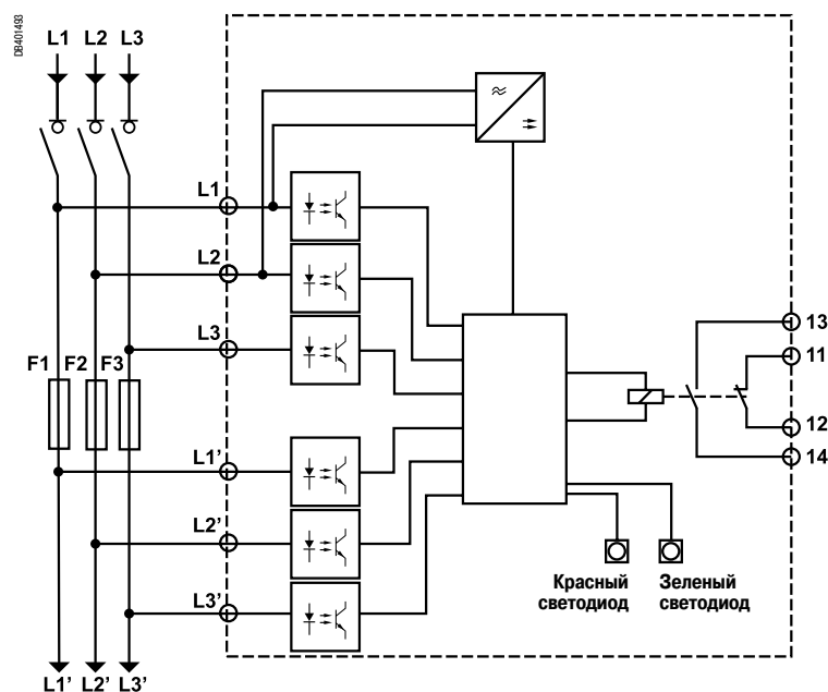
Устройство контроля состояния предохранителей в ISFT160 - 630
