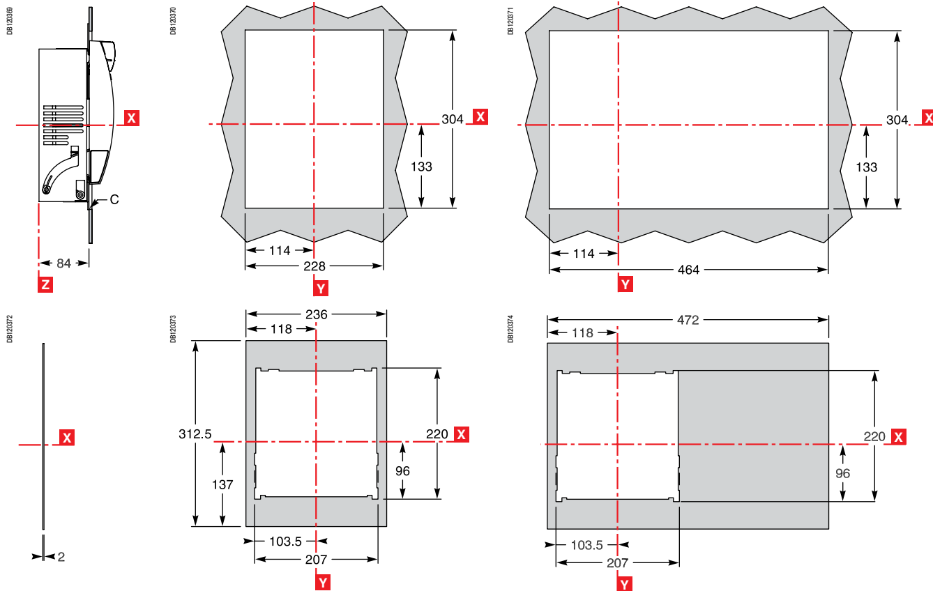
Вырез для 1 устройства
