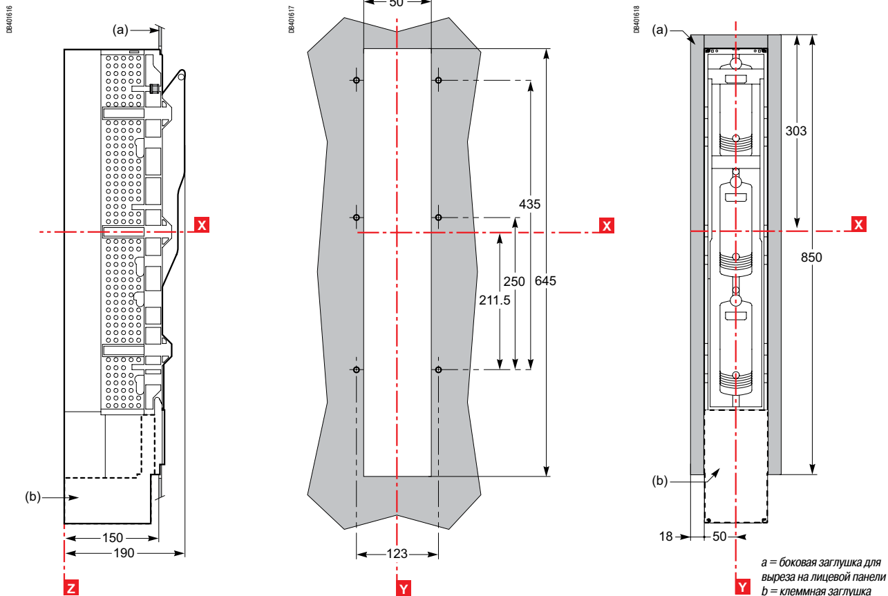
Вид спереди
