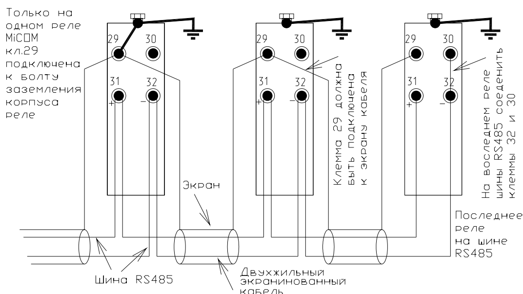
РИС. 3: ПОДКЛЮЧЕНИЕ RS485
