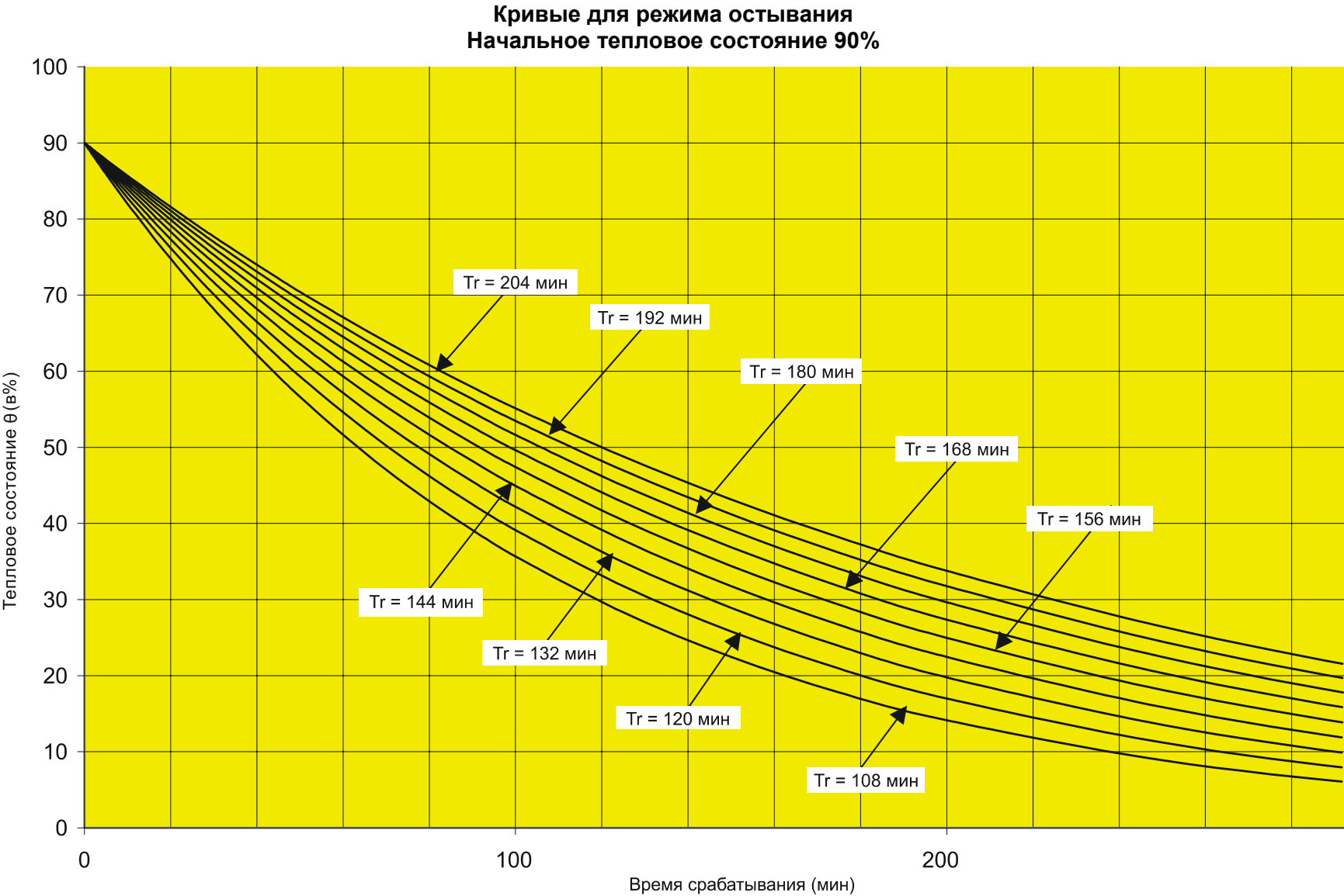
Кривые для режима остывания
