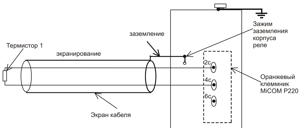
РИС. 6: ПОДКЛЮЧЕНИЕ ТЕРМИСТОРОВ
