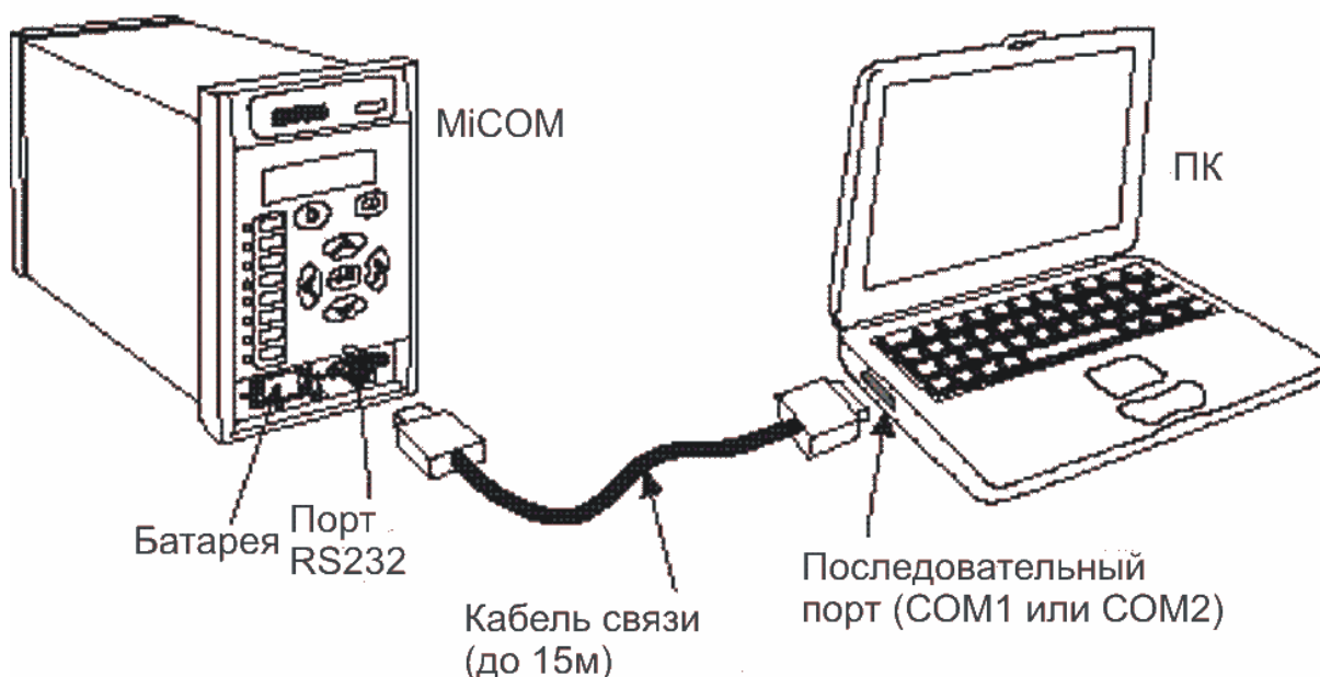
RS 232 кабель
