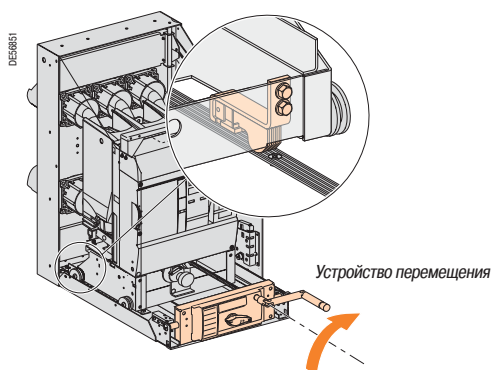
Положение «рабочее»
