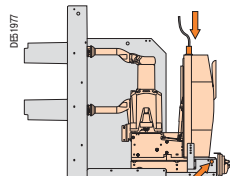
Испытательное положение
