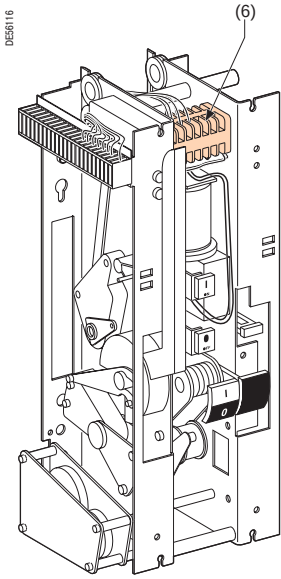
Привод выключателя
