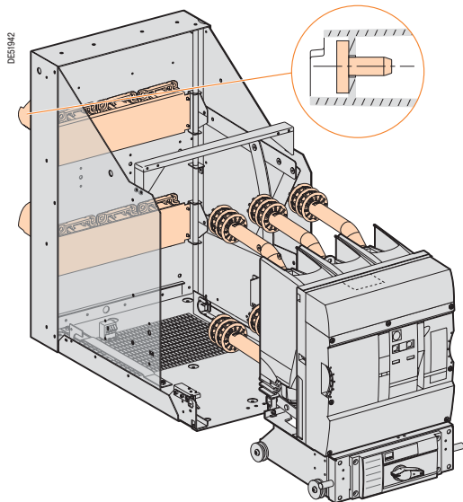
Силовая цепь
