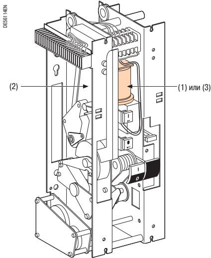
Привод
