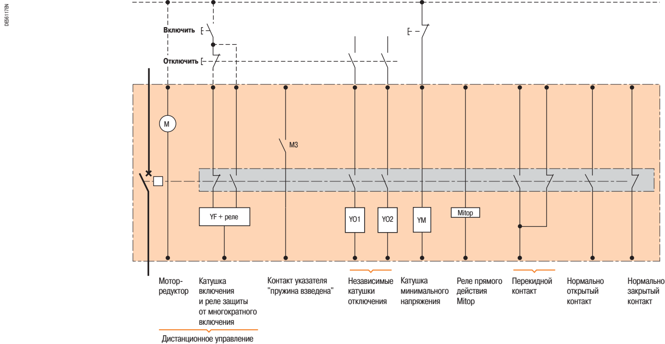
Принципиальная схема
