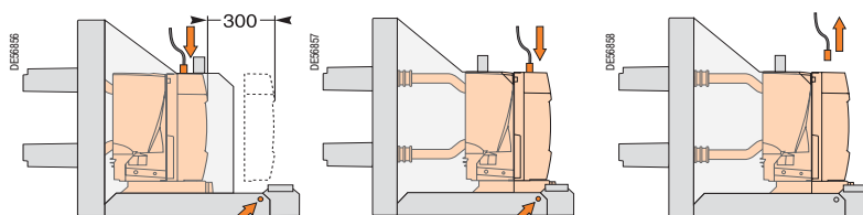
Положение «рабочее»
