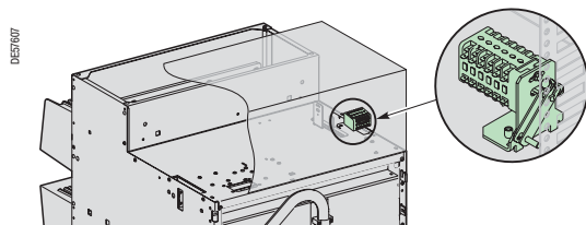
Блок - контакты
