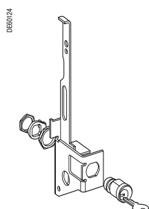
Блокировка врезным замком в отключенном положении (8)
