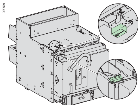
Блокировка соответствия
