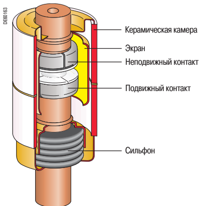
Рис. 1. Составные части вакуумной камеры выключателя
