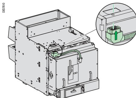
Подключение разъема низкого напряжения
