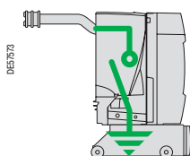
Выкатное заземление сборных шин
