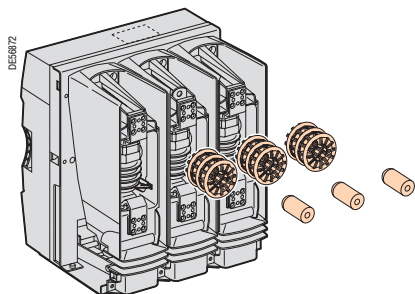
Розетки и контакты
