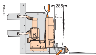
Рабочее положение
