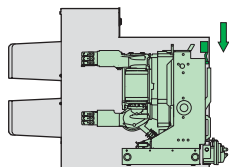
Отсоединенное положение
