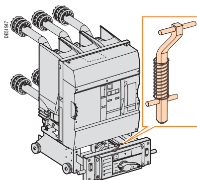
Блокировка двери отсека выключателя
