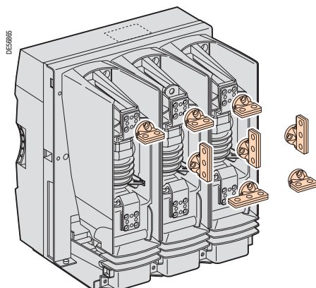
Три типа контактных площадок
