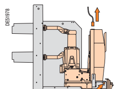
Положение "выкачен"
