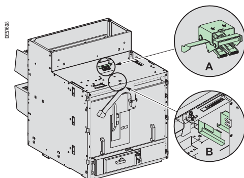
(А) Блокировка 50 кА (В) Разряд пружины привода выключателя при выкате.
