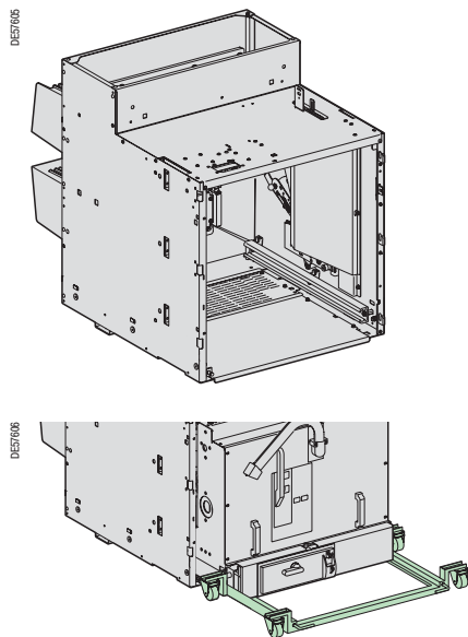
Сервисная тележка
