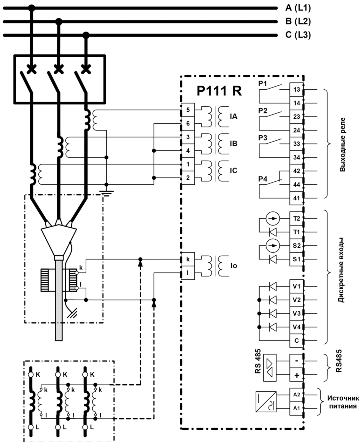
Рис. 19. Схемы подключения
