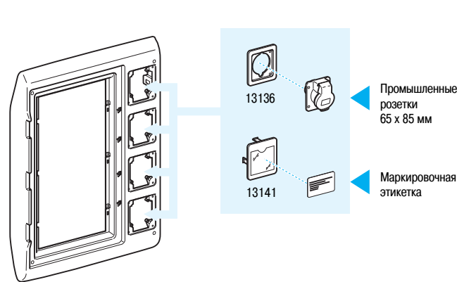
Щитки для модульных устройств с интерфейсным модулем
